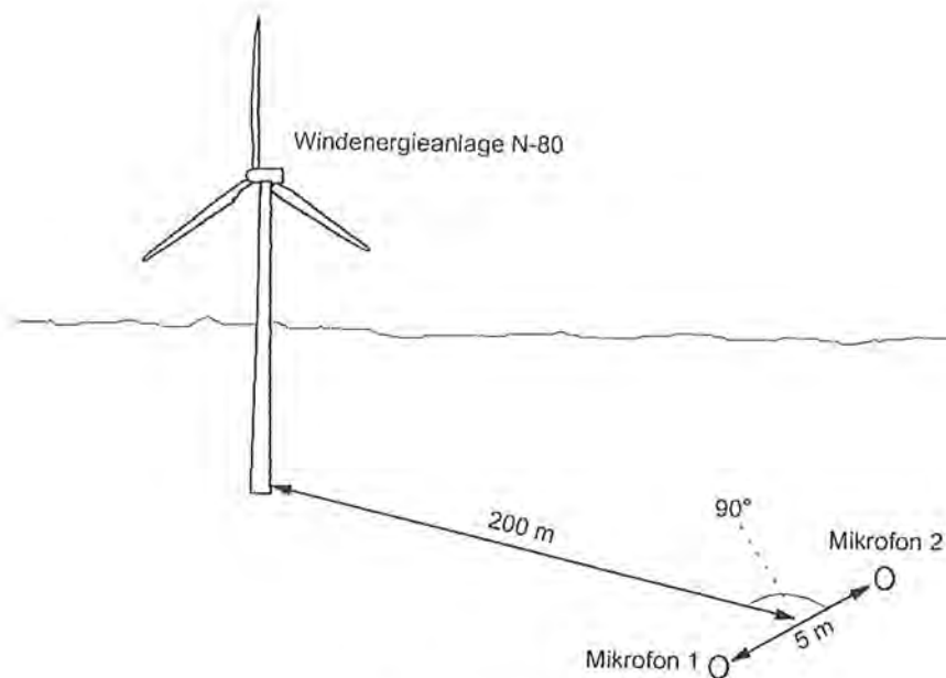
Bild 2. Skizze der Messgeometrie
