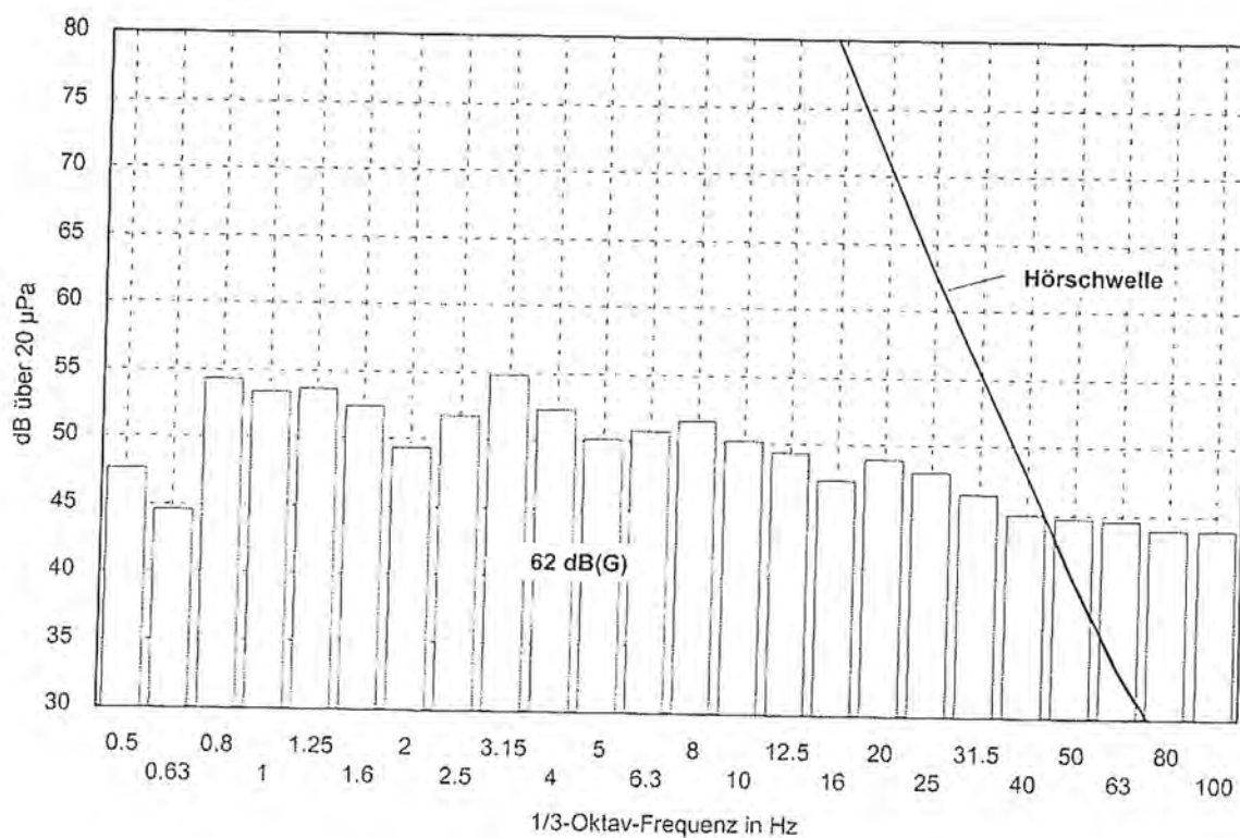
Bild 4. Typisches Terzspektrum und Hörschwelle nach DIN 45680
