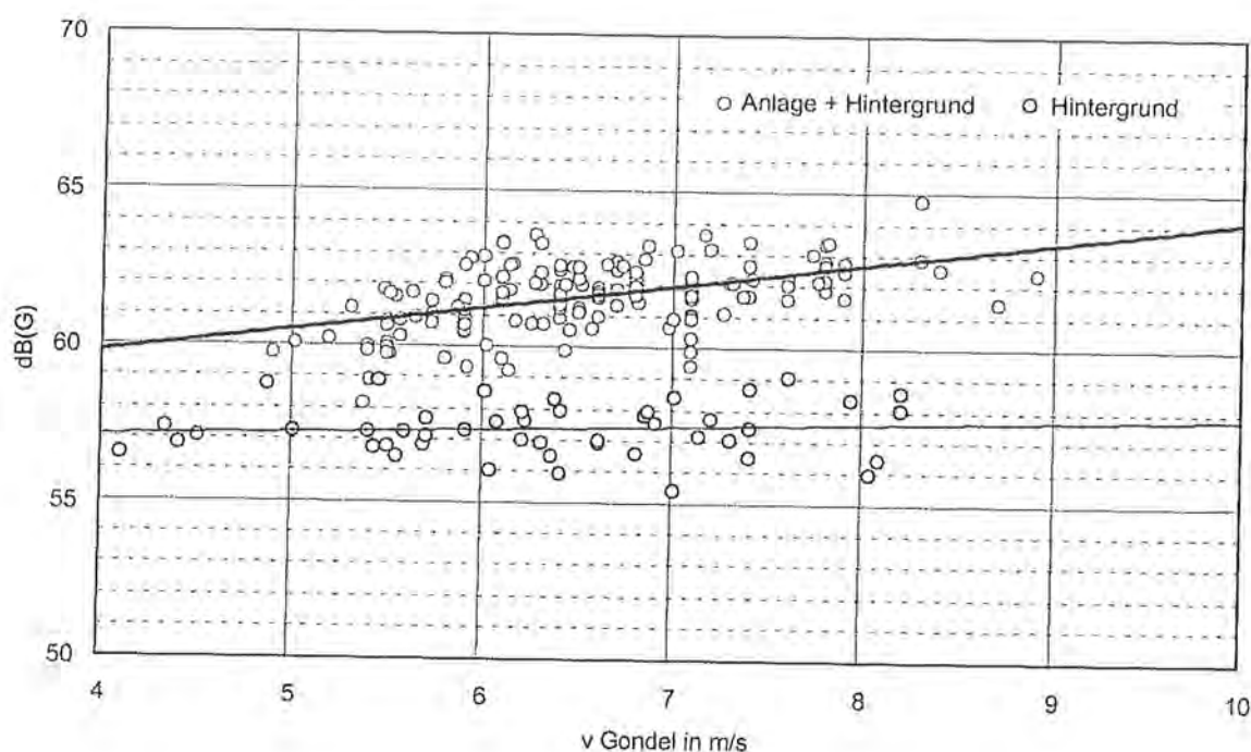
Bild 6. Gemessene G-bewertete Schalldruckpegel in Abhängigkeit von der Windgeschwindigkeit
